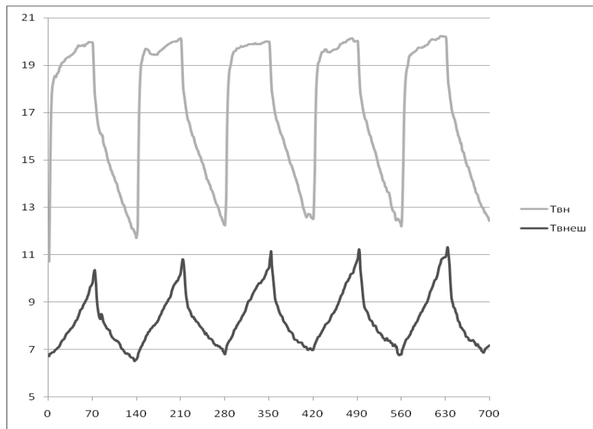
Рис. 6. Температура в торцевых сечениях регенератора inVENTer (вторая скорость).
