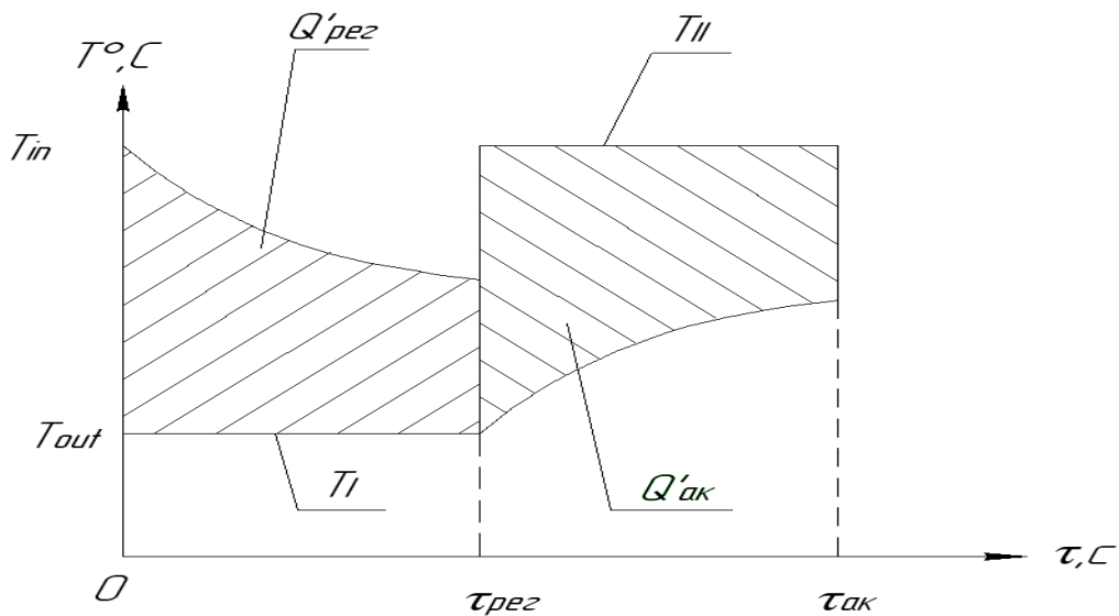
Рис.2. Изменение температуры воздуха в торцевых сечениях регенератора.
