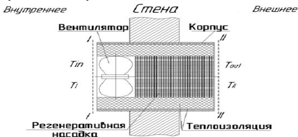
Рис.1. Конструкция СПРТ.
